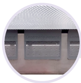
Luchtopeningen met insectengaas van ABS
