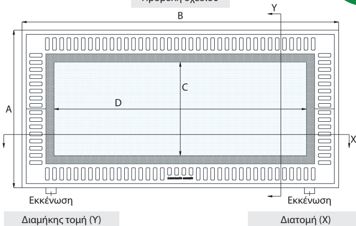
Προβολή σχεδίου
