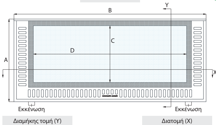
Προβολή σχεδίου
