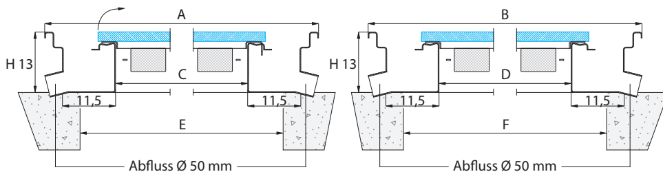
Längsschnitt (Y)
