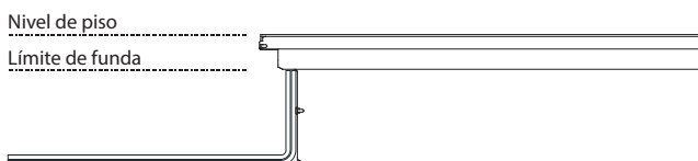
Figura D: Aplicación de la funda líquida/impermeabilizante líquido con llana.
