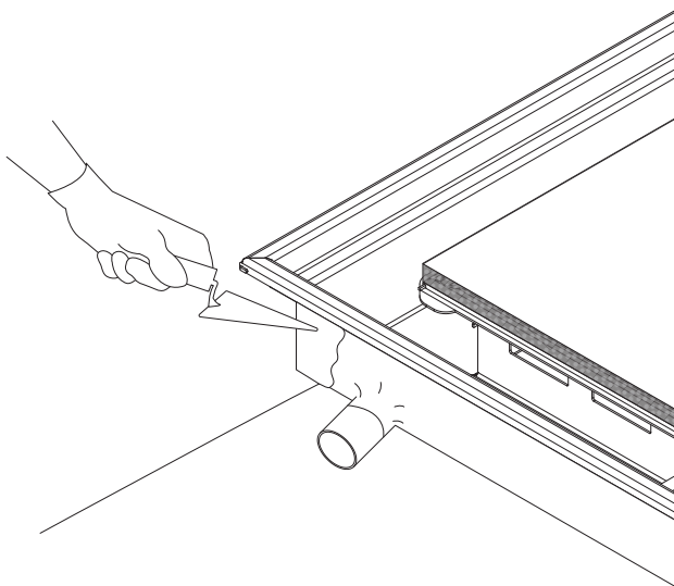
Abbildung D: Die Bitumenbahn bis zur abgebildeten Höhe verlegen.
