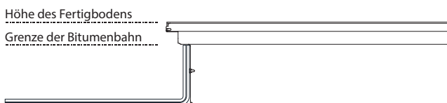
Abbildung E: Anbringung des flüssigen Dichtmittels mittels Spachtel.
