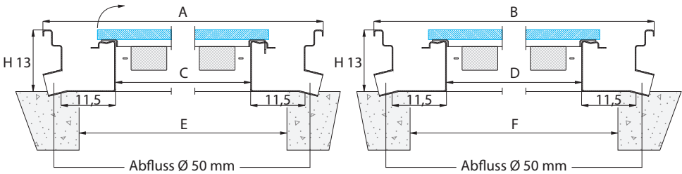
Längsschnitt (Y)
