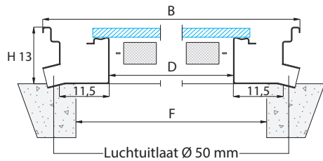
Dwarsdoorsnede (X)
