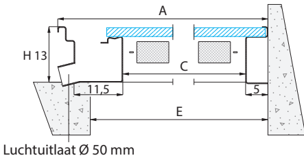
Lengtedoorsnede (Y)
