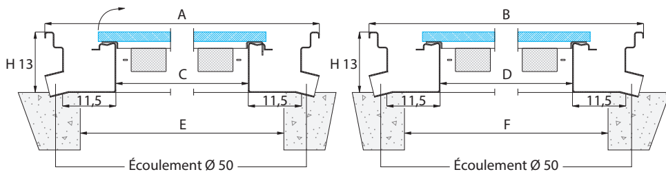
Section longitudinale (Y)
