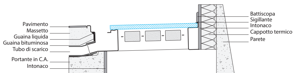
Schema di posa a ridosso di un muro
