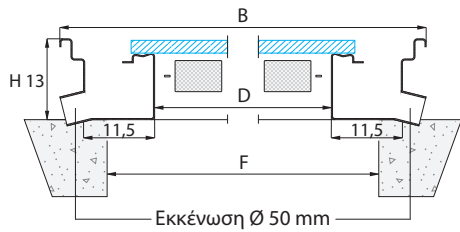
Εκκένωση \varnothing 50 mm
