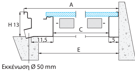
Εκκένωση \varnothing 50 mm
