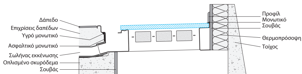
Σχέδιο τοποθέτησης κοντά σε έναν τοίχο
