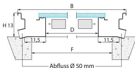
Querschnitt (X)
