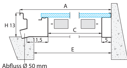
Längsschnitt (Y)
