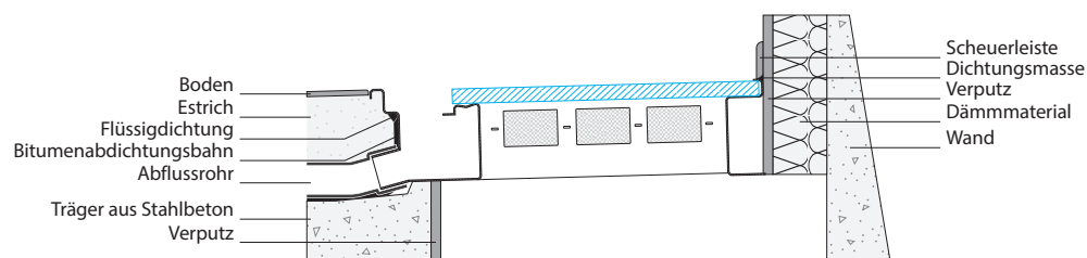
Einbauschema an einer Mauer
